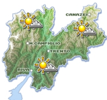
Zero termico ore 13: 800 m
