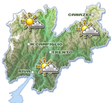
Zero termico ore 13: 900 m
