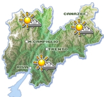
Zero termico ore 01: 800 m
