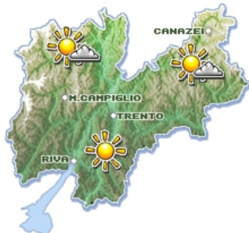
Zero termico ore 13: 1200 m
